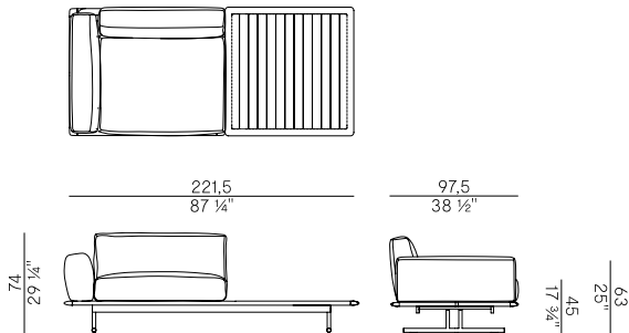
955/DT-220-OUT modulo angolare con tavolino destro o sinistro \ corner unit with right or left coffee table
