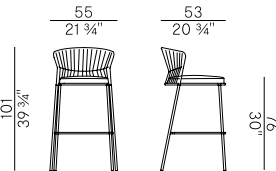
923/A sgabello alto impilabile \ stackable barstool ✚ 4 con cuscino \ with cushion ✚ 6 senza cuscino \ without cushion
