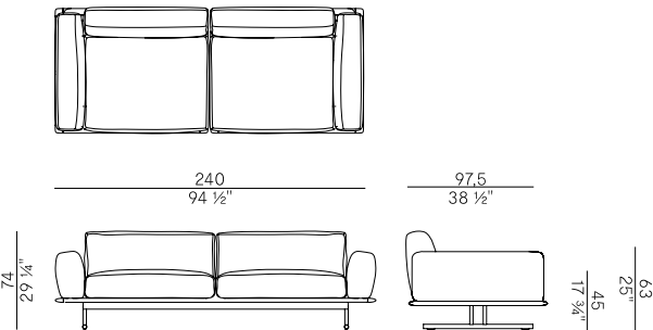
955/D-240-OUT modulo 2 posti con bracciolo destro e sinistro \ 2 seats unit with right and left armrest
