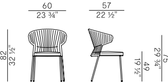
923/P-IMP poltroncina dining impilabile \ stackable dining armchair ✚ 4 con cuscino \ with cushion ✚ 6 senza cuscino \ without cushion
