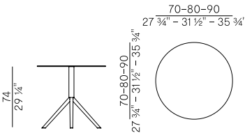
887/TC tavolo pieghevole e impilabile \ folding and stackable table
