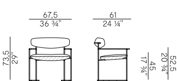
922/LMB-OUT poltrona lounge \ lounge armchair
