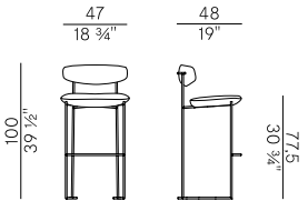
922/A-OUT sgabello alto \ barstool
