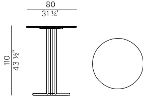
955/TAC-OUT tavolo alto \ bar table
