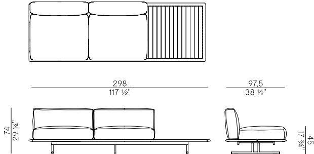
955/DT-300-OUT modulo 2 posti con tavolino destro o sinistro \ 2 seats unit with right or left coffee table
