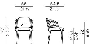
942/PAR-OUT poltroncina pozzetto \ tub chair
