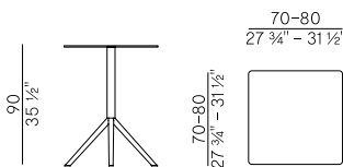
887/TSQ tavolo pieghevole e impilabile \ folding and stackable table
