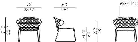
698/LP poltrona lounge impilabile \ stackable lounge armchair ×4 cuscino \ cushion
