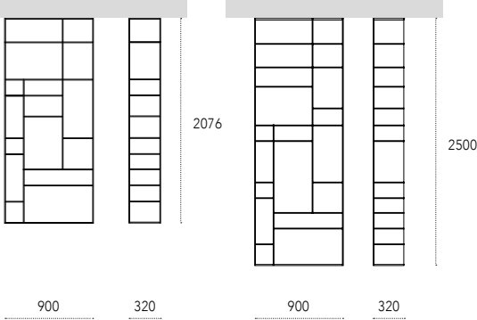
Dimensioni - Dimensions (mm) Levia Air
