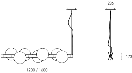
Dimensioni - Dimensions (mm) Sundown Round orizzontale - horizontal
