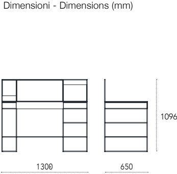
Dimensioni - Dimensions (mm)
