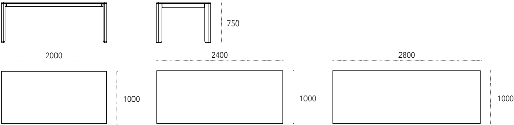
Dimensioni - Dimensions (mm)
