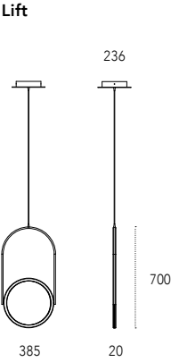
Dimensioni - Dimensions (mm)
