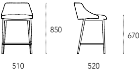
Dimensioni - Dimensions (mm) Sgabello basso - Low stool
