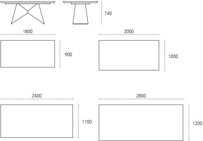
Dimensioni - Dimensions (mm) Piano rettangolare - Rectangular top
