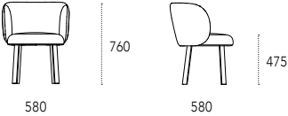
Dimensioni - Dimensions (mm)
