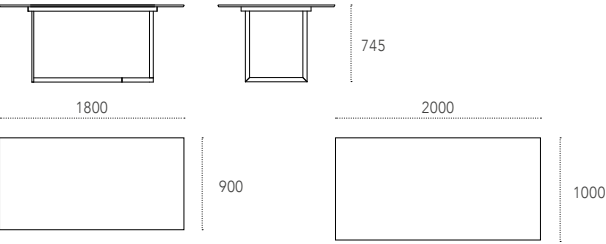
Dimensioni - Dimensions (mm)
