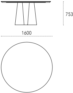
Dimensioni - Dimensions (mm) Piano in vetro o legno - Glass or wood top
