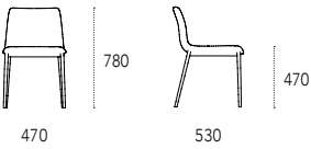
Dimensioni - Dimensions (mm)
