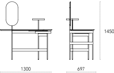
Dimensioni - Dimensions (mm) Mira Beauty
