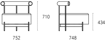
Dimensioni - Dimensions (mm) Poltrona - Armchair
