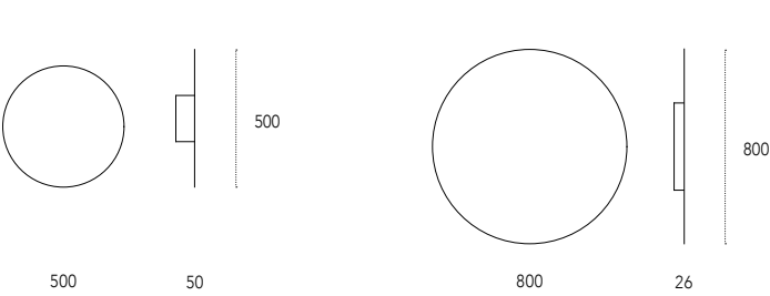
Dimensioni - Dimensions (mm)
