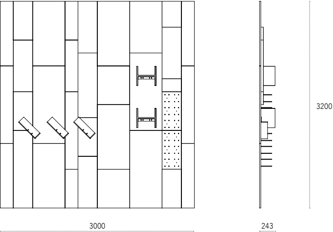
Dimensioni - Dimensions (mm)
