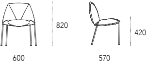
Dimensioni - Dimensions (mm)
