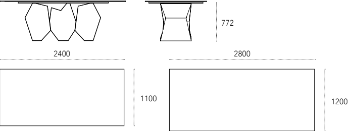
Dimensioni - Dimensions (mm) Piano rettangolare - Rectangular top
