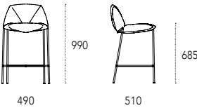
Dimensioni - Dimensions (mm) Sgabello basso - Low stool
