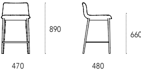
Dimensioni - Dimensions (mm) Sgabello basso - Low stool
